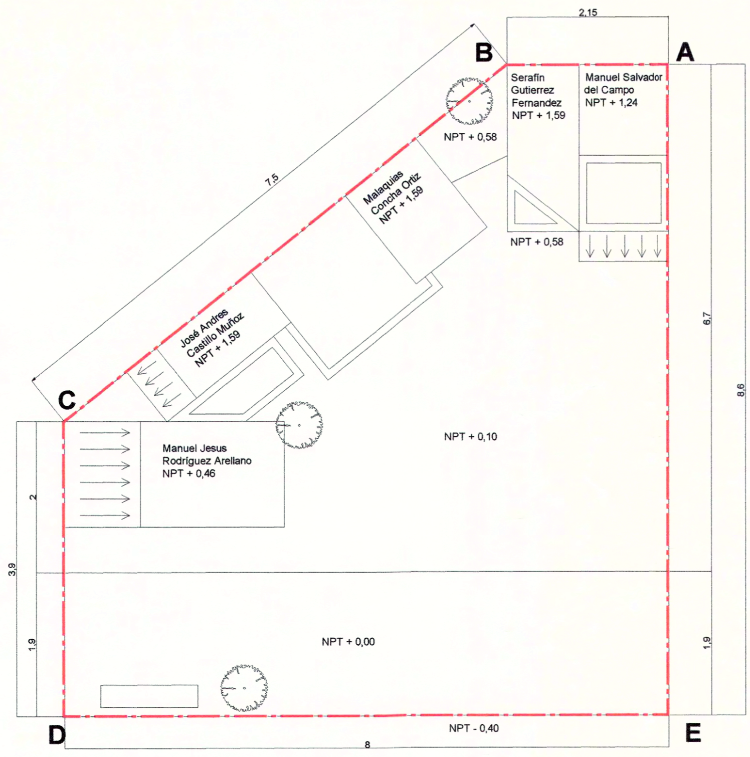
PLANO DE LÍMITE MONUMENTO HISTÓRICO PATIO DE HOMBRES ILUSTRES Esc. 1/50
