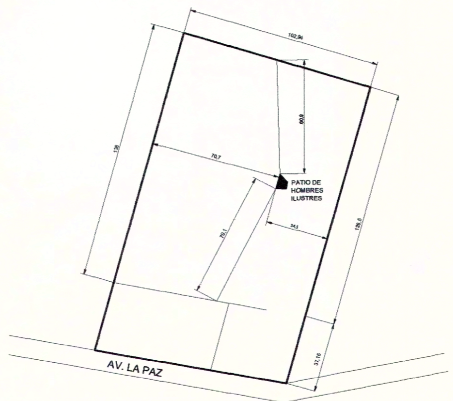
PLANO DE EMPLAZAMIENTO CEMENTERIO DE VILLA ALEGRE Esc. 1/2000
