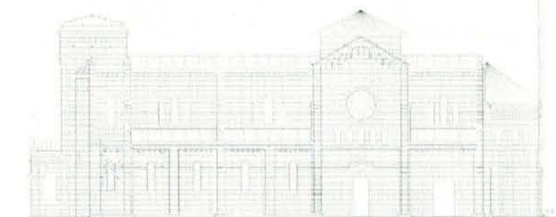
ELEVACIÓN SUR
