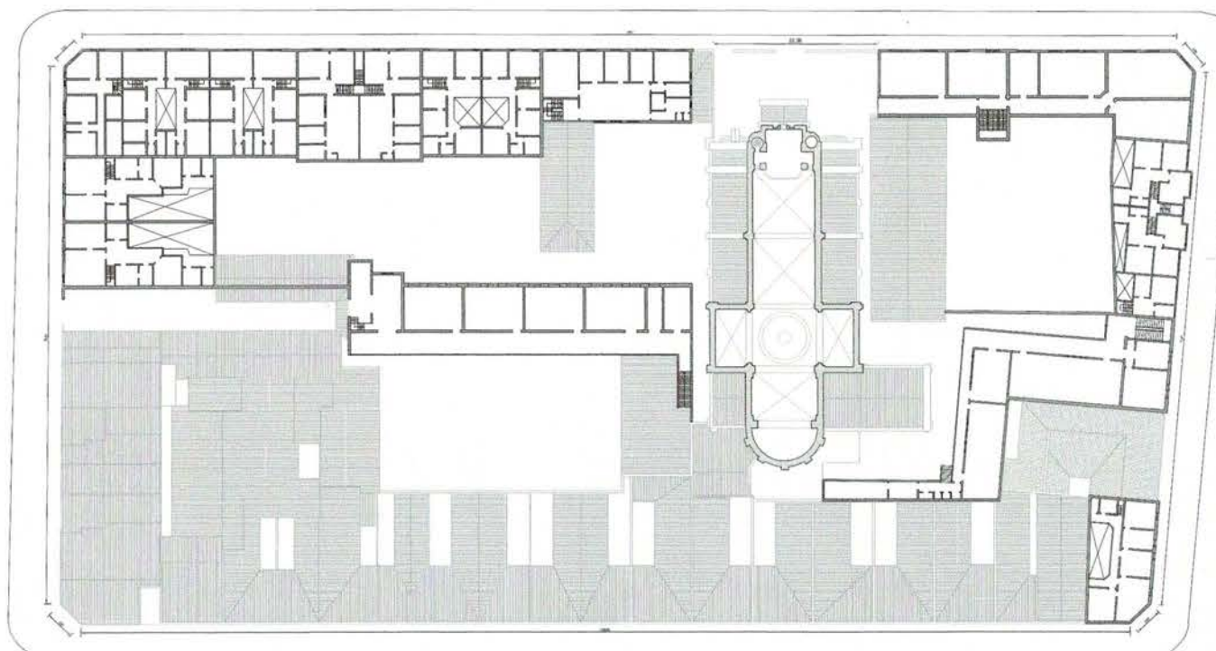
PLANTA GENERAL 2º PISO DEL CONJUNTO
